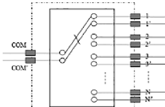
■ Duplex 1xN
